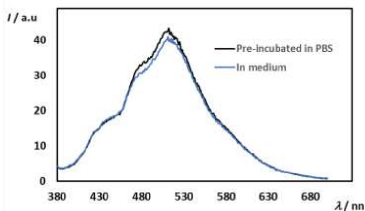
شکل ۴- طیف نشر لوسیجین آزاد شده از کمپلکس CX4-LCG انکوبه شده در بافر فسفات و رهایش در محیط کشت (منحنی مشکی) و یا انکوباسیون و رهایش در محیط کشت (منحنی آبی).
