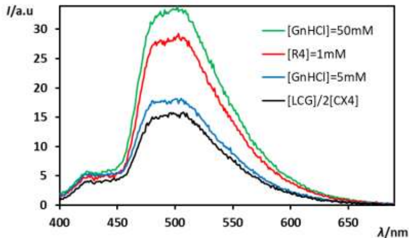
شکل ۳- طیف نشر فلورسانس سنجش جایگزینی نشانگر. آزاد شدن لوسیجین از کمپلکس CX4-LCG توسط جایگزینی با آنالیت‌های پپتید تترآرژنین R4 و گوانیدین هیدروکلرید (Gn-HCl) با افزایش نشر فلورسانس همراه است.
