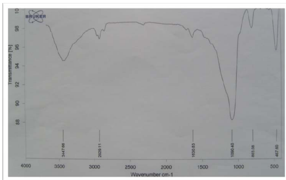
شکل ۲- طیف FT-IR پیگمان اصلی. باندهای جذبی ویژه پلی ان های ایزوپروپنوئید به خوبی قابل مشاهده است.
