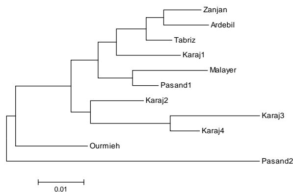
شکل ۳- دندروگرام ۱۱ جمعیت علف باغ حاصل از مقادیر داده‌های فاصله ژنتیکی باروش Neighbor-joining.
