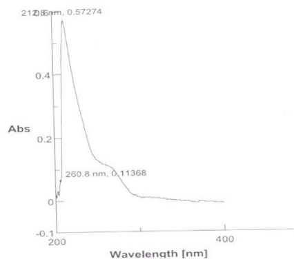
نمودار ۸-۱- طیف مربوط به IMHP در نمونه تیمار شده در روز سوم بعد از تلقیح (حذف دیازینون و افزایش IMHP)
