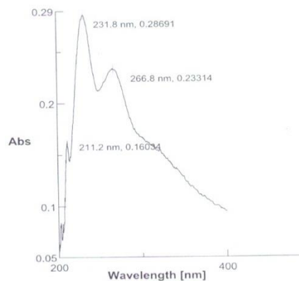
نمودار ۵-۱- طیف مربوط به دیازینون و IMHP (در حال تشکیل)
