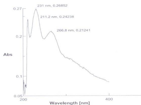
نمودار ۷-۱- طیف مربوط به دیازینون و IMHP در نمونه تیمار شده
