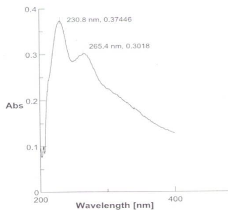
نمودار ۱-۳- طیف دیازینون با \lambda_{max}=230nm مربوط به نمونه شاهد در روز پنجم
