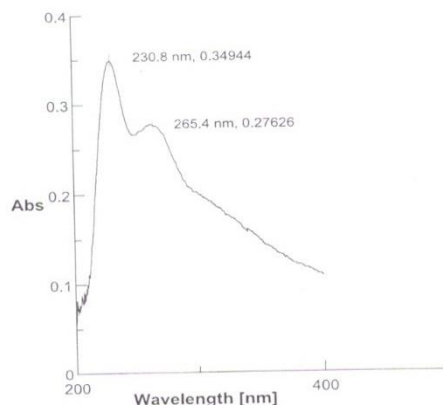
نمودار ۴-۱- طیف مربوط به دیازینون در نمونه تیمار شده
