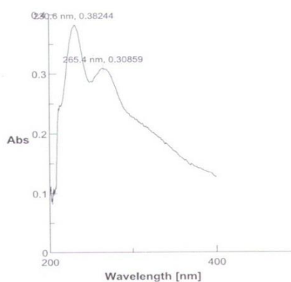
نمودار ۱-۲- طیف دیازینون با \lambda_{max}=230nm مربوط به نمونه شاهد در روز اول
