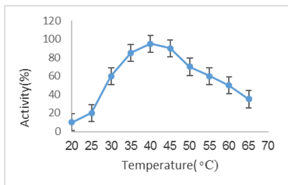
نمودار ۱۰- اثر دما بر فعالیت آنزیم OPH
