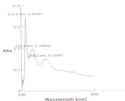
نمودار ۶-۱- طیف مربوط به دیازینون و IMHP در نمونه تیمار شده
