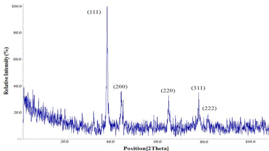
شکل ۲- الگوی تفرق اشعه ایکس نانوذرات نقره در شرایط بهینه سنتز. الگوی پیکهای XRD مربوط به ساختار مکعبی مراکز سطحی (fcc) Face-centered cubic (centered cubic) (۱۱۱)، (۲۰۰)، (۲۲۰)، (۳۱۱) و (۲۲۲) در طیف نمونه نقره دیده می‌شود. زوایای \theta ۲ مربوط به الگوی نقره در ۴۴/۵، ۳۸/۰۴، ۶۴، ۷۷/۷، ۸۱/۷ دیده می‌شود.
