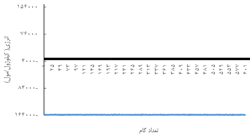
نمودار ۲- همگرایی انرژی طول شبیه‌سازی در سیستم شامل پاکلی تاکسول + یک آستروپسین A
