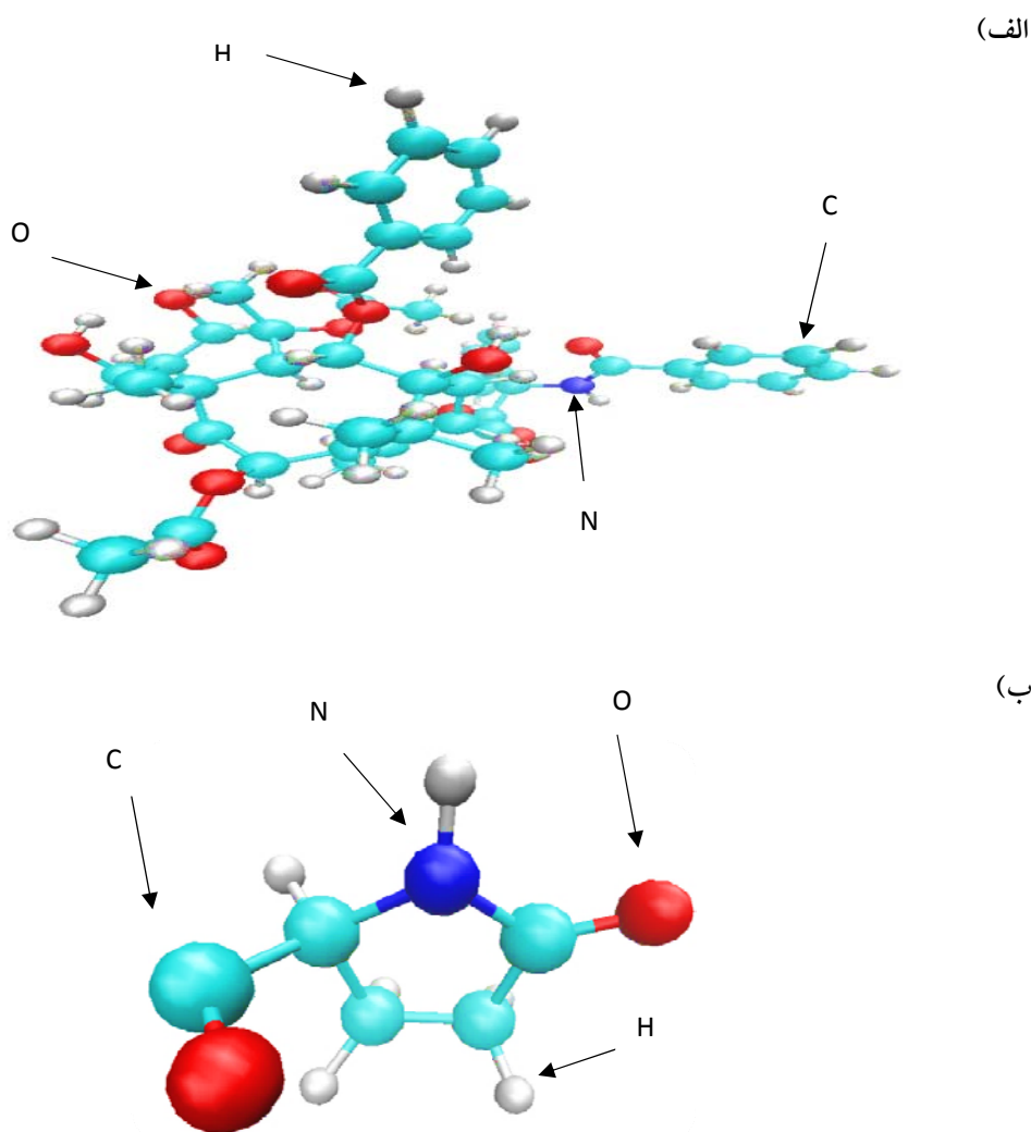
شکل ۲- ساختار بیهینه شده الف) مولکول پاکلی تاکسول ب) زنجیر جانبی اسید آمینه مولکول آستروپسین A
