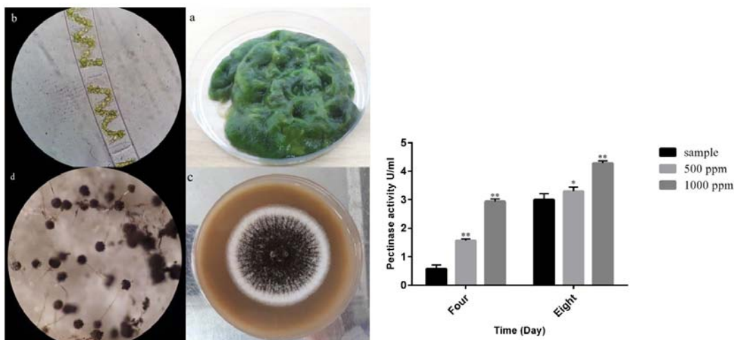
شکل ۲- (a) تصویر میکروسکوپی توده رشته ای جلبک Spirogyra sp. (b). تصویر درشت نمایی شده میکروسکوپ نوری از ریشه جلبک Spirogyra همراه با کلروپلاست ماریپیچی (c). تصویر میکروسکوپی از هیف و اسپوره های قارچ A. niger روی محیط کشت PDA. (d). تصویر درشت نمایی شده میکروسکوپ نوری قارچ A. niger
