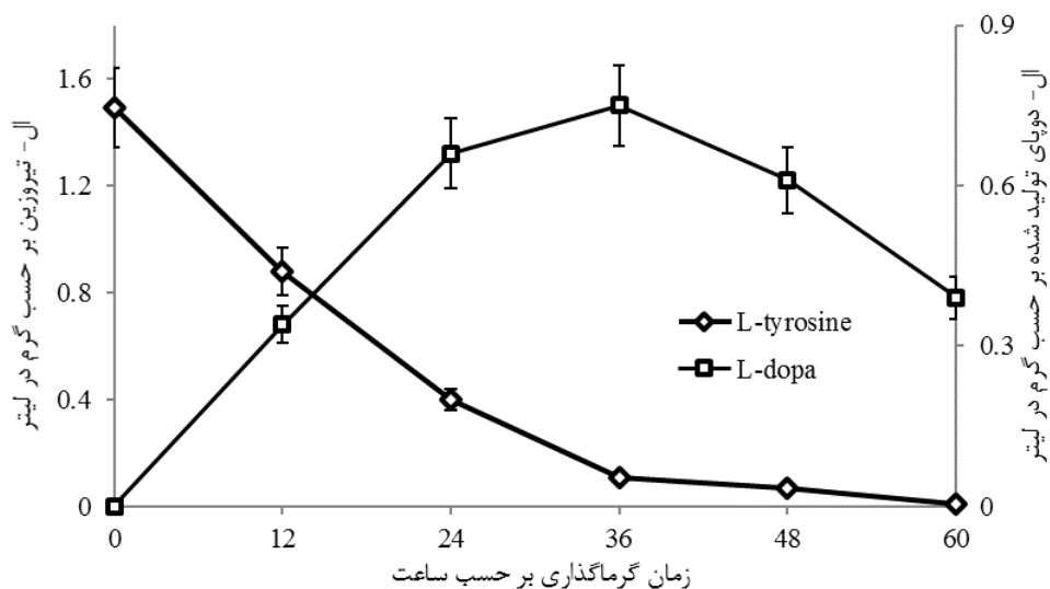
شکل ۵- زی تبدیل ال-تیروزین به ال-دوپا بوسیله سلولهای در حال استراحت Halobacillus sp. SL-7 تحت شرایط بهینه شده توسط روش تک فاکتوری. نتایج ارائه شده میانگین سه بار آزمایش و با \pm 1 معرف انحراف معیار است.
