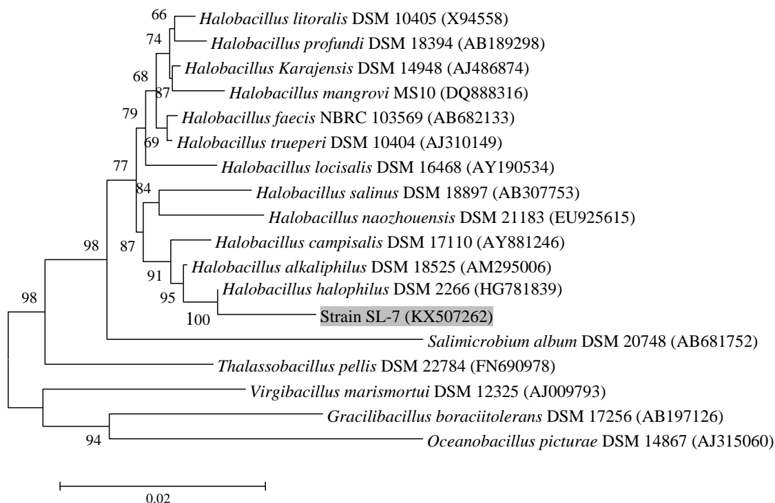
شکل ۳- درخت فیلوژنی سویه‌ی SL-7 و دیگر اعضای جنس Halobacillus بر اساس ژن تکثیر یافته‌ی rDNA ۱۶S. شماره دسترسی سویه‌های ثبت شده در پراپتور آورده شده است.
