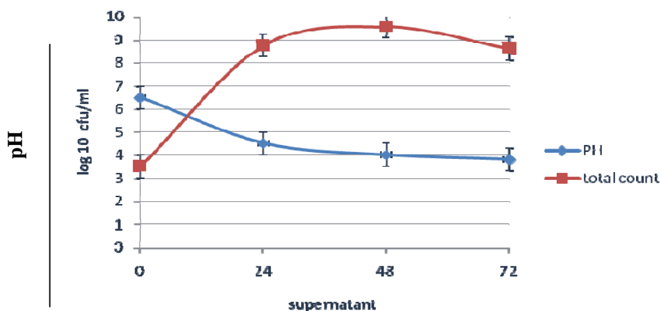
شکل ۱ - تغییرات pH و total count در مدت زمان ۷۲ ساعت از کشت باکتری Bifidobacterium bifidum در محیط آبگوشت MRS در دمای ۳۷ درجه سانتی گراد (اعداد گزارش شده میانگین ۳ نمونه اندازه گیری شده است).
