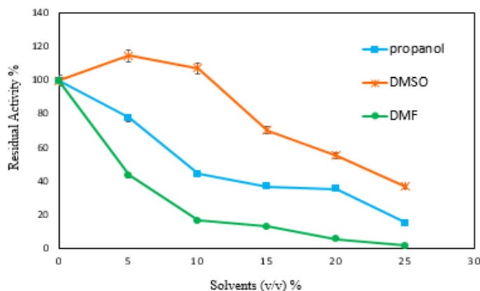
شکل ۳- فعالیت اندوگلوکاناز AaCel9A در حضور حلالهای DMSO, DMF و پروپانول
