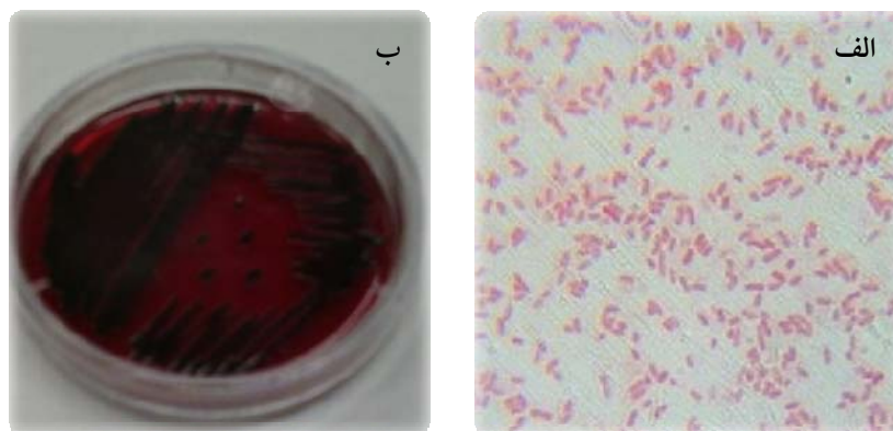
شکل ۲- کلنی‌های سیاه رنگ رشد کرده در سطح محیط کشت کلیگر آگار (الف) و تصویر میکروسکوپی سلول‌های میله‌ای شکل و گرم منفی رنگ‌آمیزی شده به روش گرم (ب) جدایه ME1 (بزرگمایی ۱۰۰۰ برابر).
