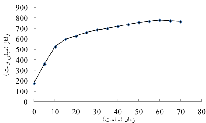
شکل ۴- منحنی ولتاژ مدار باز جدایه ME1 در پیل سوختی میکروبی در دمای ۳۰ درجه سانتی‌گراد.
