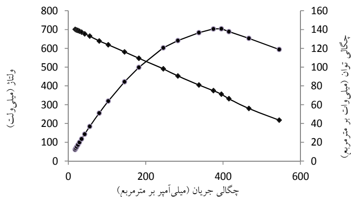
شکل ۵- منحنی قطبیت و چگالی توان برحسب چگالی جریان. (◆) ولتاژ (میلی‌ولت)، (●) توان (میلی‌وات).
