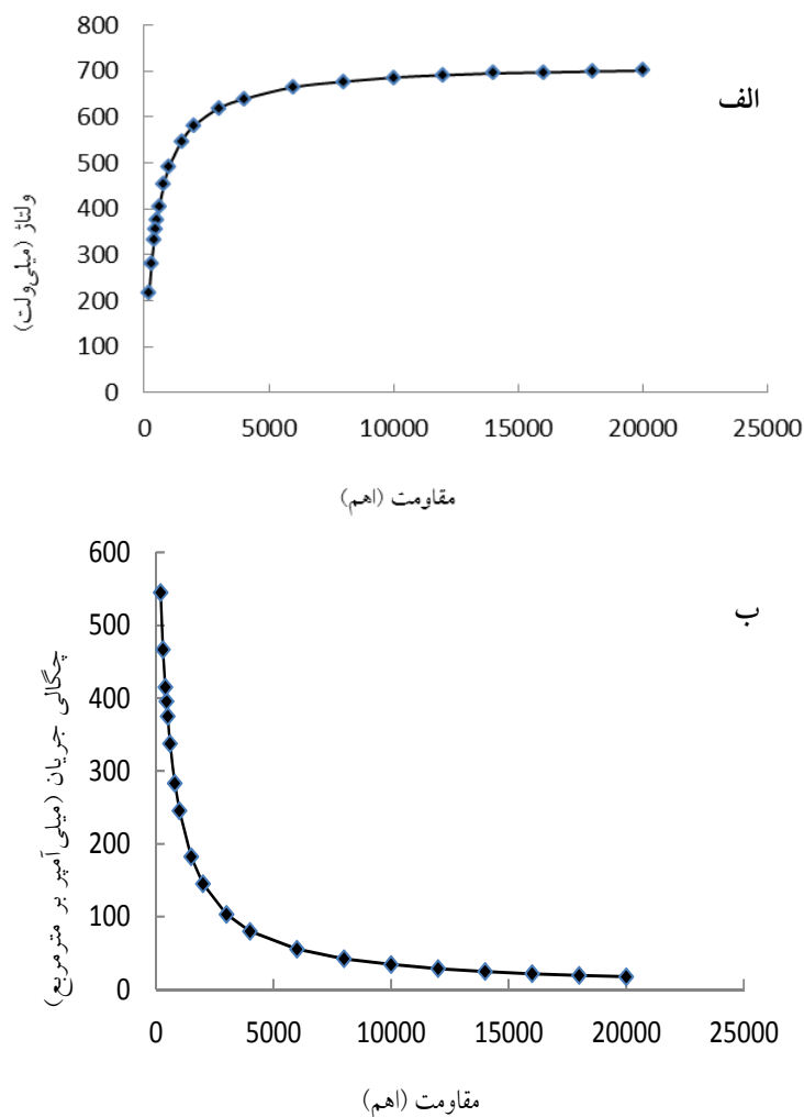
شکل ۶- ارتباط بین مقاومت با ولتاژ (الف) و مقاومت با چگالی جریان (ب).
